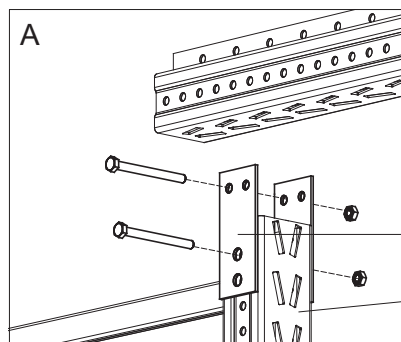
СТОЙКА 70 UPRIGHT 70
