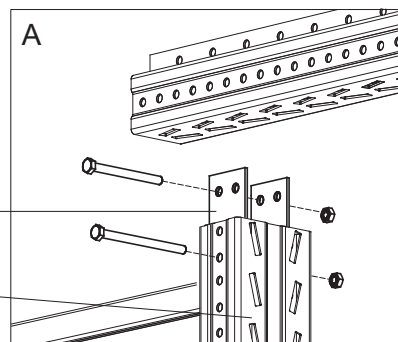
СТОЙКА 85, 100, 120 UPRIGHT 85, 100, 120
